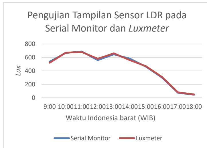
Gambar 6 Diagram Garis Pengujian Tampilan sensor LDR pada serial monitor dan Luxmeter
